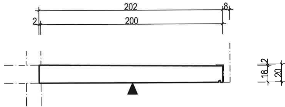
COUPE A Ech: 1/25
